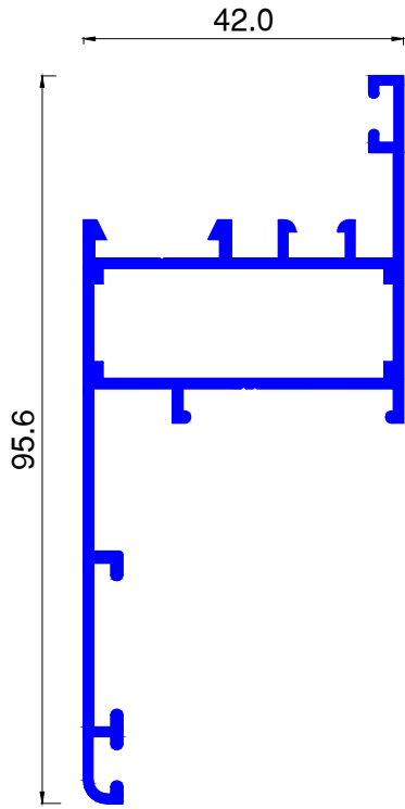
ALU421 kg/ml 0.913
