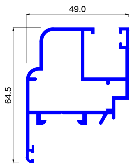
ALU436 kg/ml 1.013
