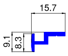
ALU325 kg/ml 0.108
