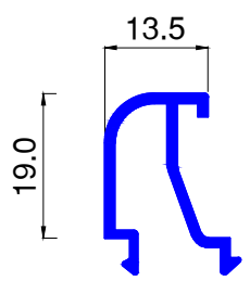
ALU325 kg/ml 0.108
