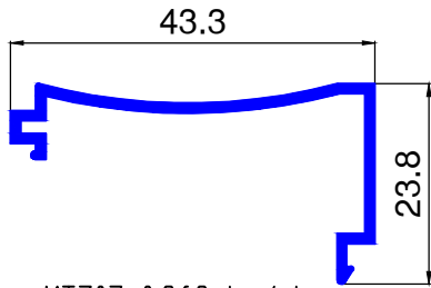
MT707 0.262 kg/ml.
