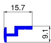
ALU325 Kg/ml. 0.108
