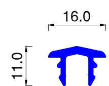
ALU730 Kg/ml. 0.140
